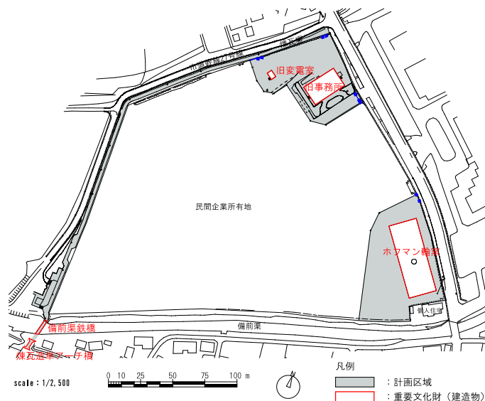
図. 2-12 位置図 (位置図は国土地理院『基礎地図情報』を利用して作成)
