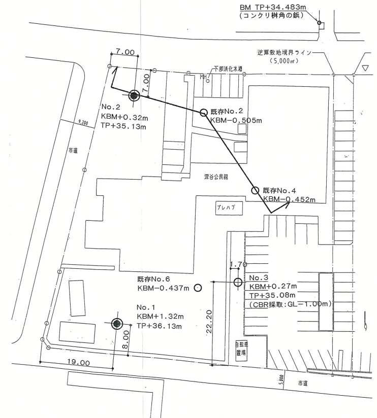
断面位置図
