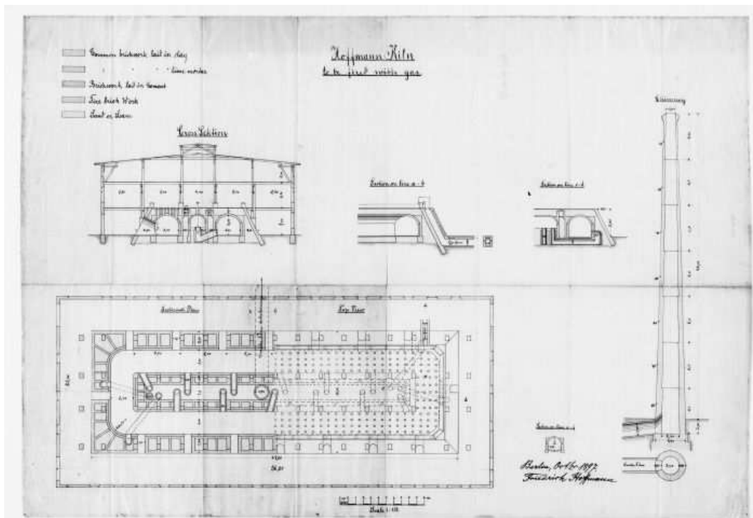
五号窯原図（明治30年）
