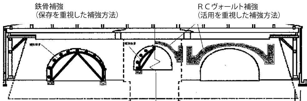
図2 補強模式図
