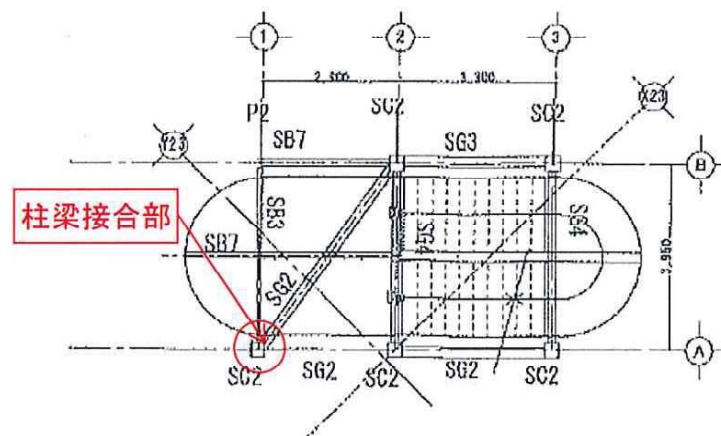
1FL+6,500 スライダー用階段構造伏図（Bスライダー階） S=1/100
