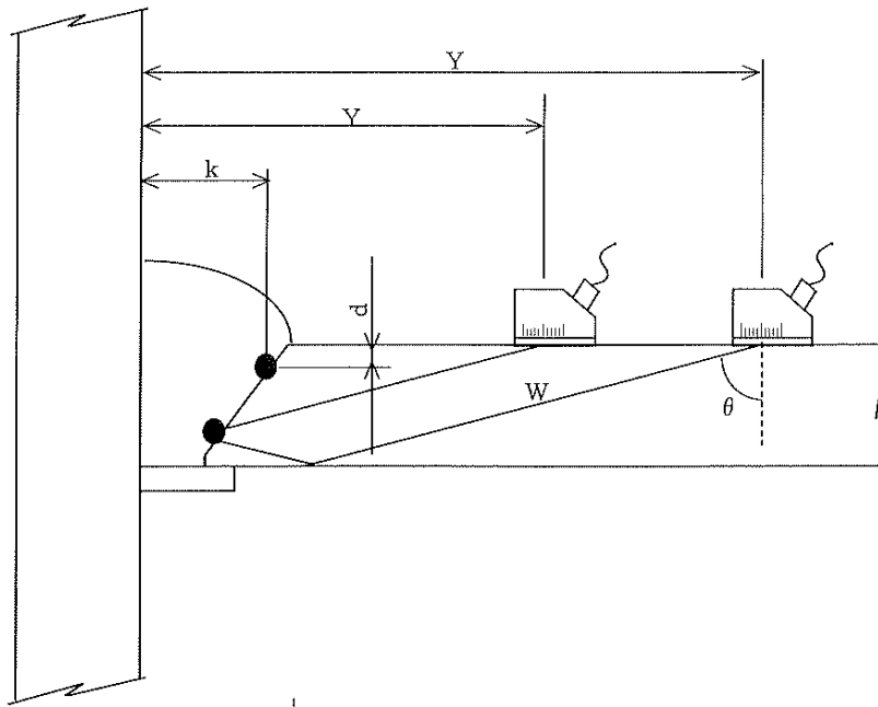
T継手
