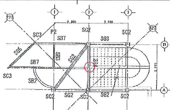
1FL+3,274 スライダ用階段構造伏図 (スロープ接続部) S=1/100
