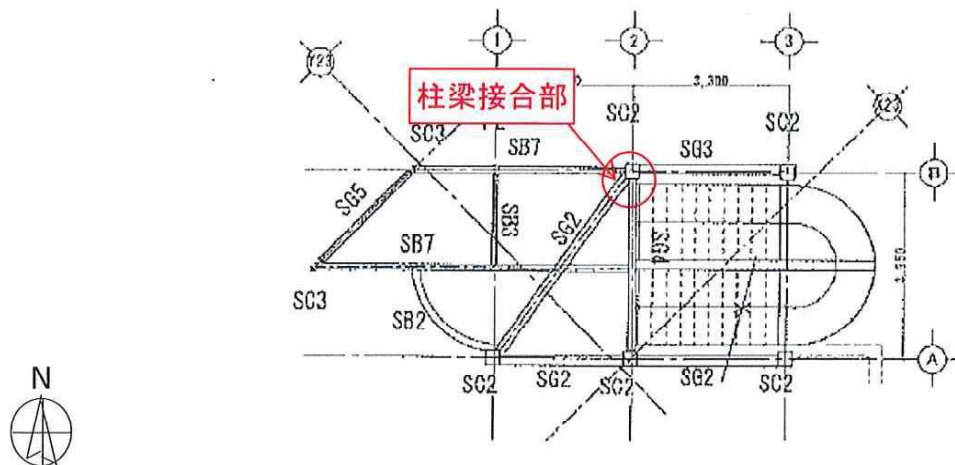
1FL+3,274 スライダー用階段構造伏図（スロープ接続階） S=1/100
