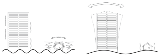
【短周期地震動】 【長周期地震動】 ▲建物の揺れやすい周期 (固有周期) は高さや構造などによって異なり、一般的に高いビルほど長い固有周期をもちます。
