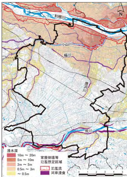
想定最大規模降雨による洪水想定図
