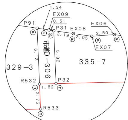
詳細図 1/250
