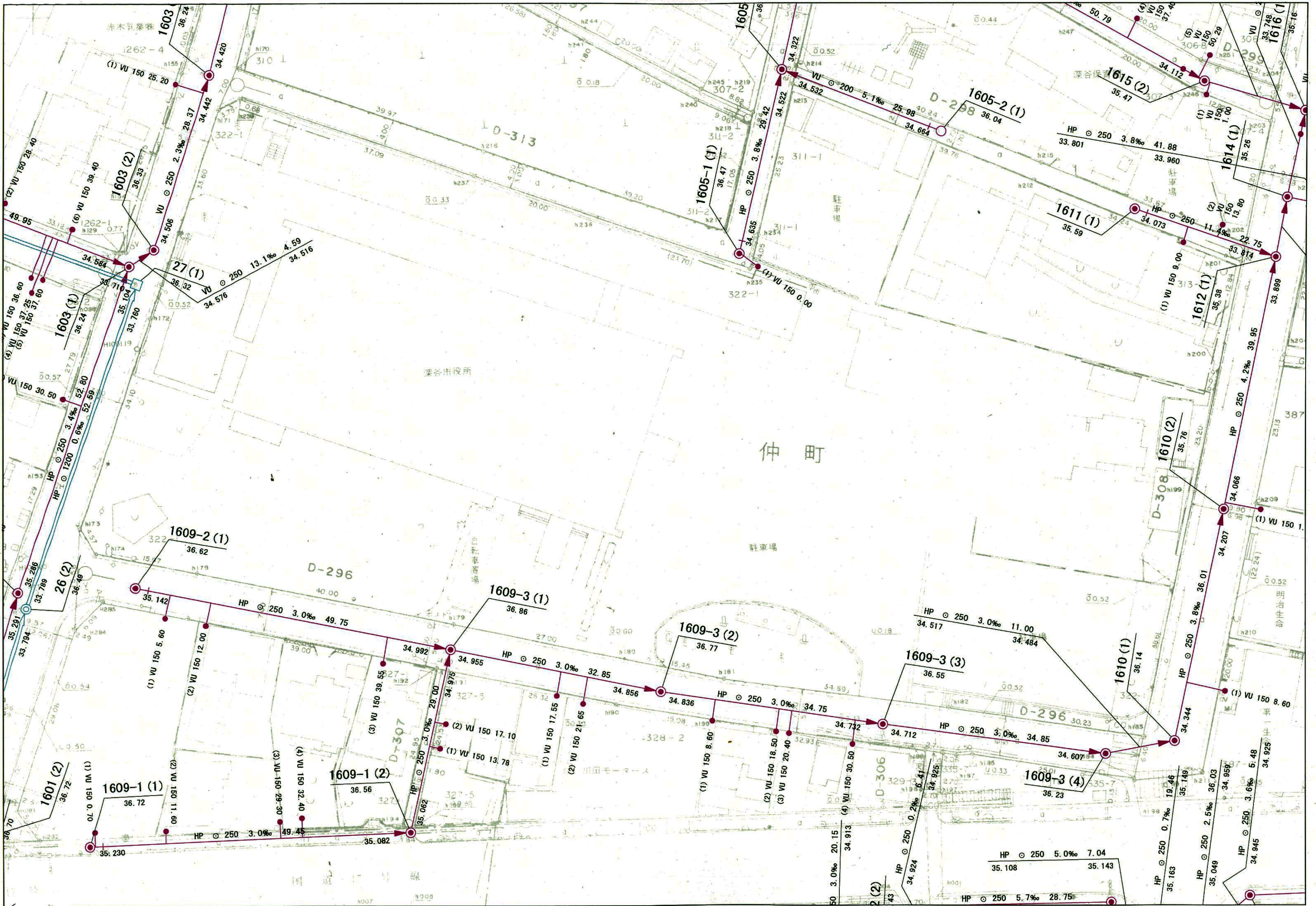
下水道台帳
