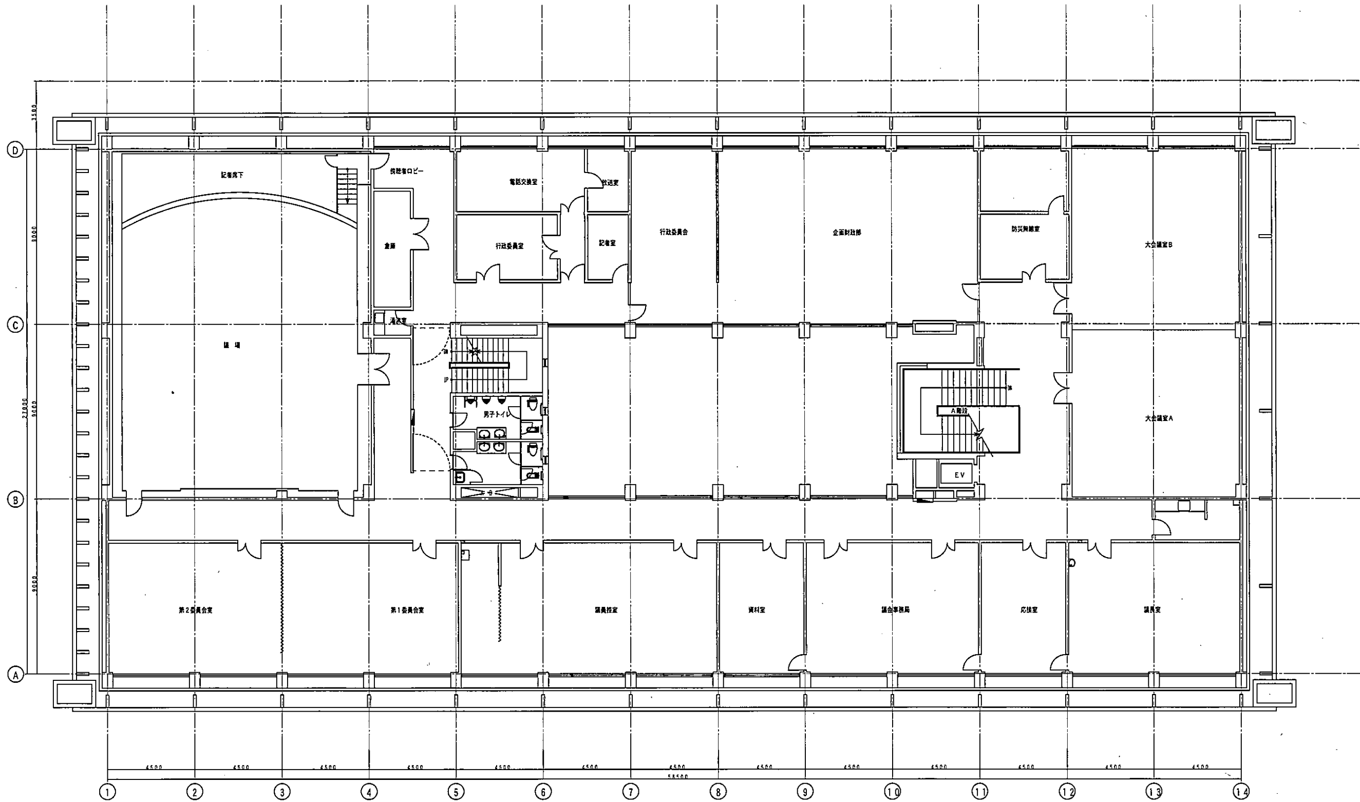
3階平面図
