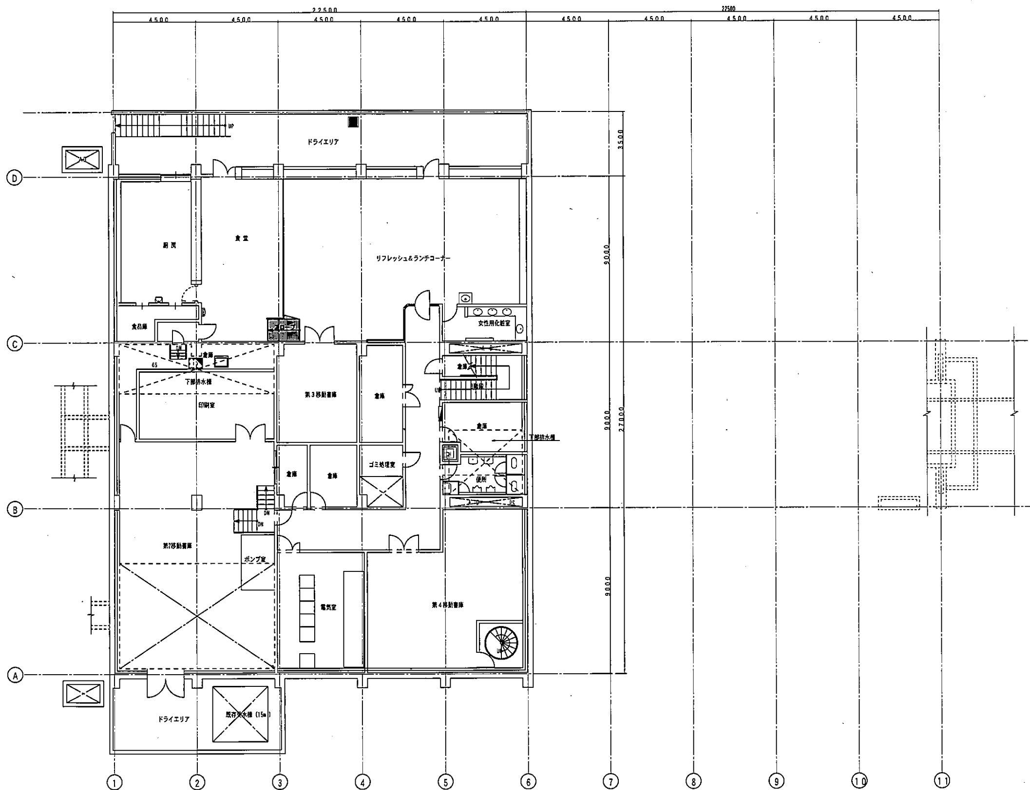
B1 階平面図
