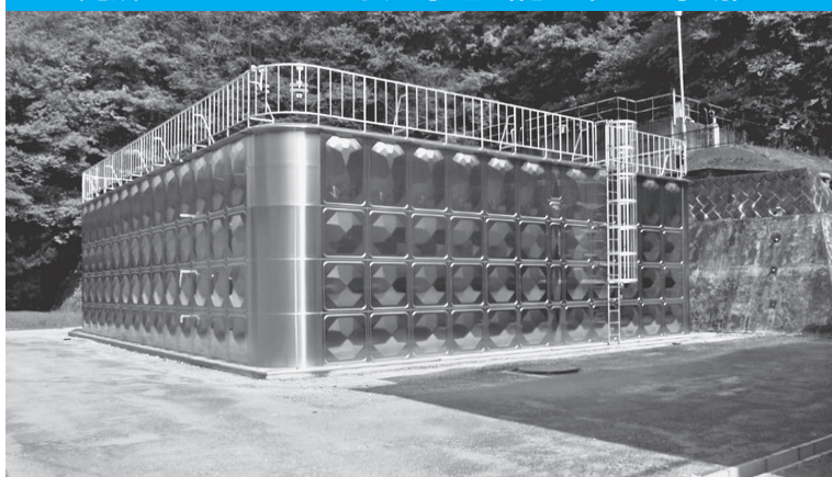
完成したステンレス製配水池（花園第二配水場）
