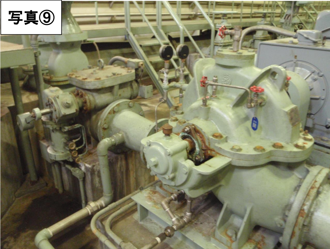
管理棟 配水ポンプ室内部配管劣化状況
