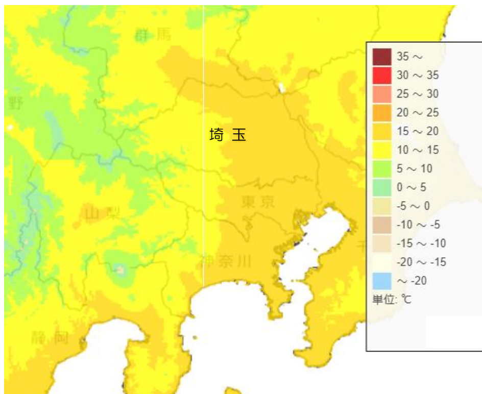
図4-7 このまま対策を行わなかった場合の埼玉県の将来の平均気温（2080～2100年）
