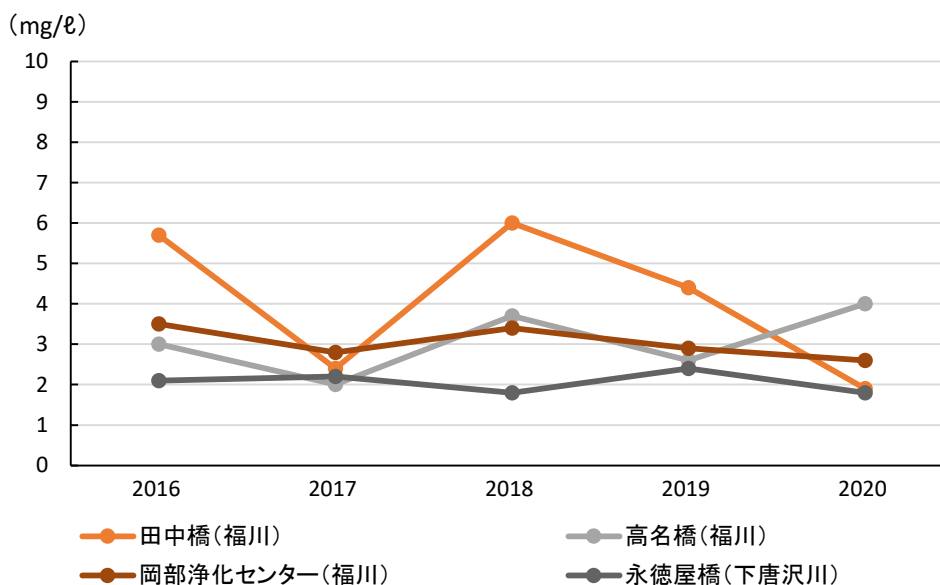
図 環境基準適用河川の年度別BOD平均値
